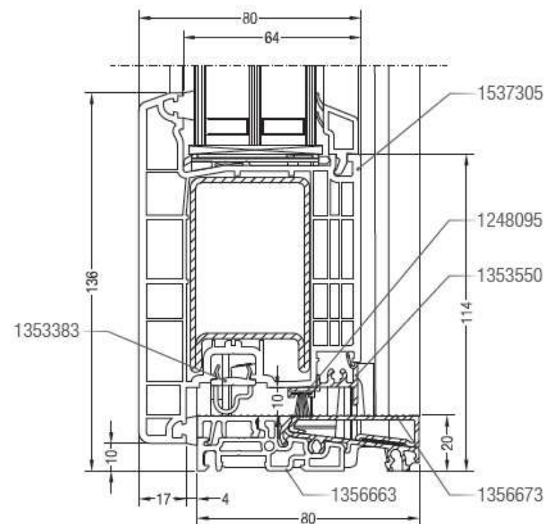
Sezione nodo anta dritta da 126 mm e soglia in Al Apertura esterna
