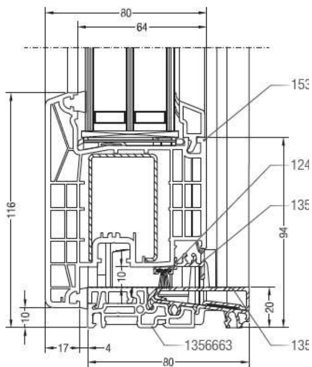
Sezione nodo anta dritta da 206 mm e soglia in Al Apertura esterna
