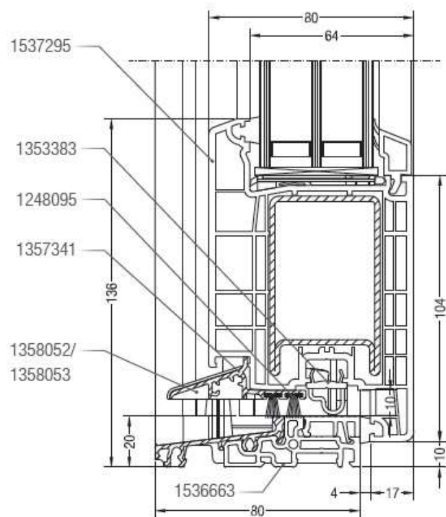
Sezione nodo anta dritta da 304 mm e soglia in Al Apertura interna
